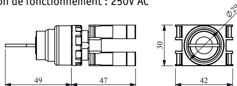
Dimensions de montage \varnothing 22,4 \pm 0,2 mm
