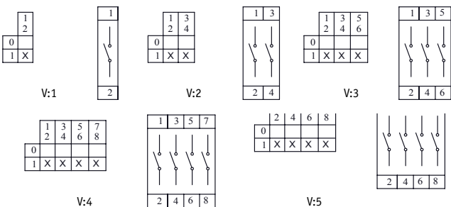
Schéma de contact
