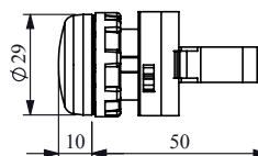
Dimension de montage Ø22,4 ±0,2 mm
